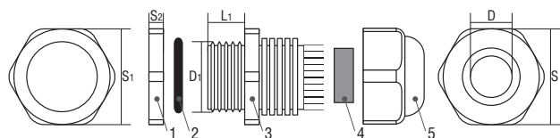
Фиксирующая гайка 1, уплотнитель 2, корпус 3, прокладка 4, гайка уплотнения 5.
